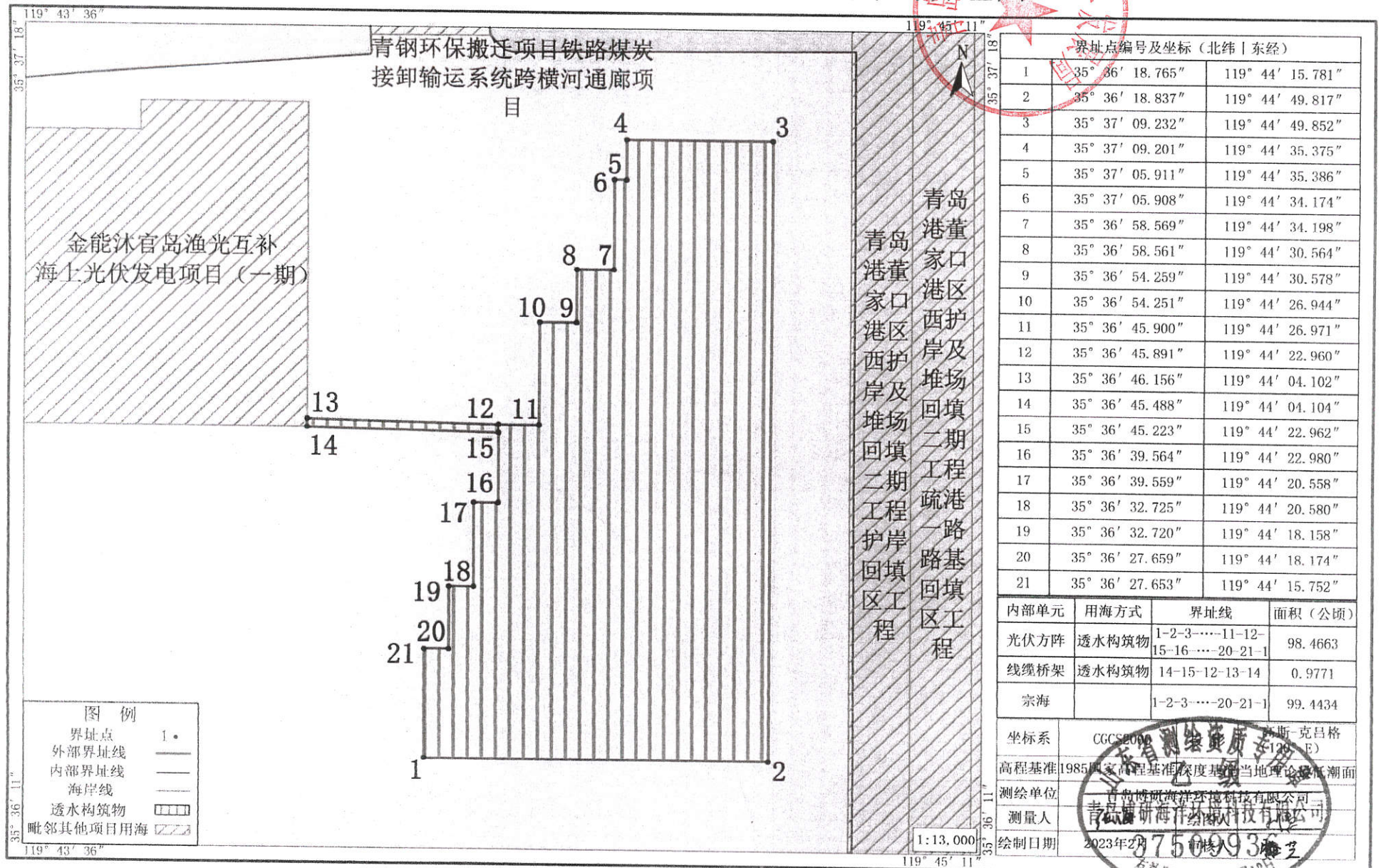
金能沐官岛海上光伏发电二期项目宗海界址图
